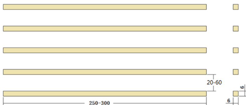
图5 跨栏示意图
