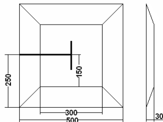
图2 锥台尺寸（mm）
