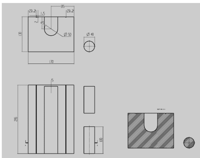
图4 管道槽和管道示意图
